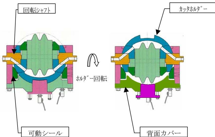
【トンネル掘進時】
