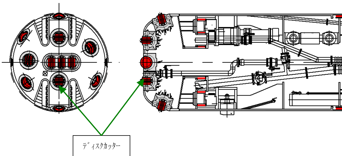
岩盤掘削シールドマシン
